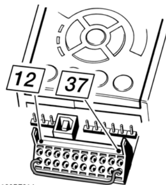
Рисунок 2.1: Соедините переключкой клемму 37 и источник напряжения 24 В=.
