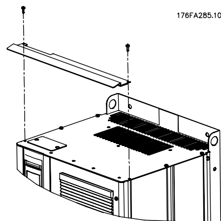
Рисунок 3.27: Установка защитной накладки.
