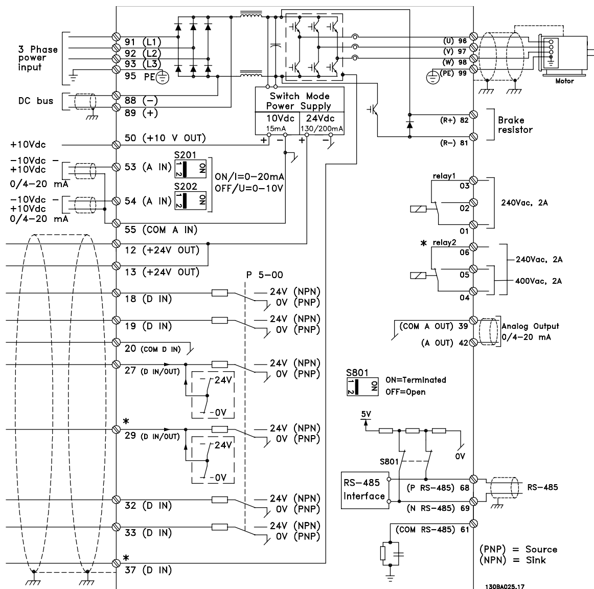
Рисунок 3.53: На схеме показаны все электрические клеммы без дополнительных устройств.
