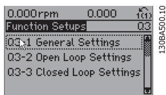
Рисунок 8.4: Шаг 4: Появляется меню настройки функций. Выберите Q3-1 Общие настройки. Нажмите [OK].
