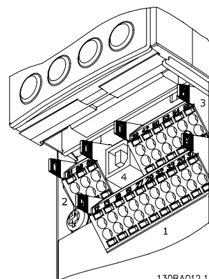
Рисунок 5.39: Клеммы управления (все корпуса)
