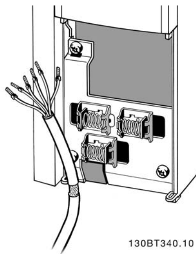
Рисунок 5.40: Зажим кабеля управления.
