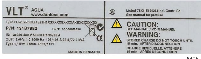
Рисунок 3.1: Пример идентификационной таблички привода VLT AQUA
