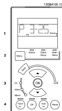
Рисунок 7.1: Цифровая панель местного управления (NLCP)
