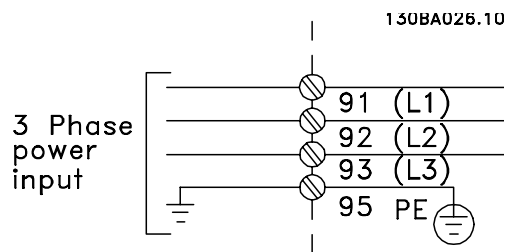
Рисунок 5.1: Клеммы сетевого питания и заземления.
