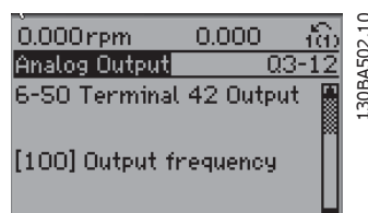
Рисунок 8.6: Шаг 6: Выберите параметр 6-50 Клемма 42, выход. Нажмите [OK].
