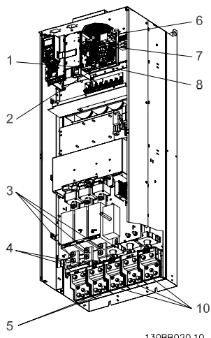
Рисунок 3.45: Compact IP 00 (Шасси) с разъединителем, плавким предохранителем и фильтром ВЧ-помех, размер корпуса E2
