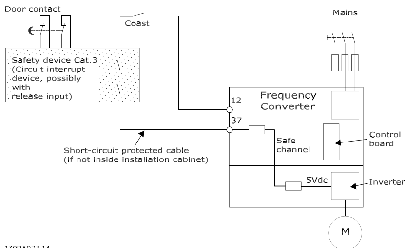
Рисунок 2.2: Рисунок, поясняющий основные особенности установки, необходимые для осуществления останова категории 0 (EN 60204-1), отвечающего требованиям категории безопасности 3 (EN 954-1).
