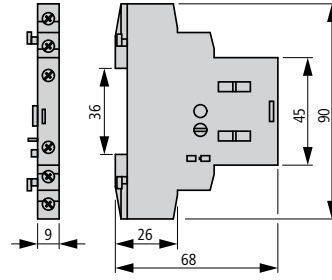
Стандартные вспомогательные контакты NHI...-PKZ... NHI...-PKZ0
