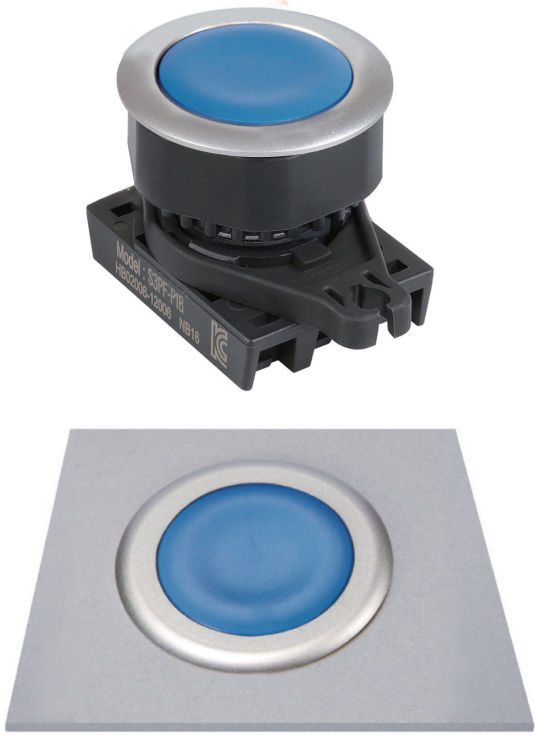
• Для монтажных отверстий - Ø30,5 мм
