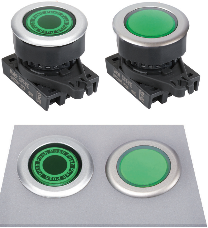
• Для монтажных отверстий - Ø30,5 мм
